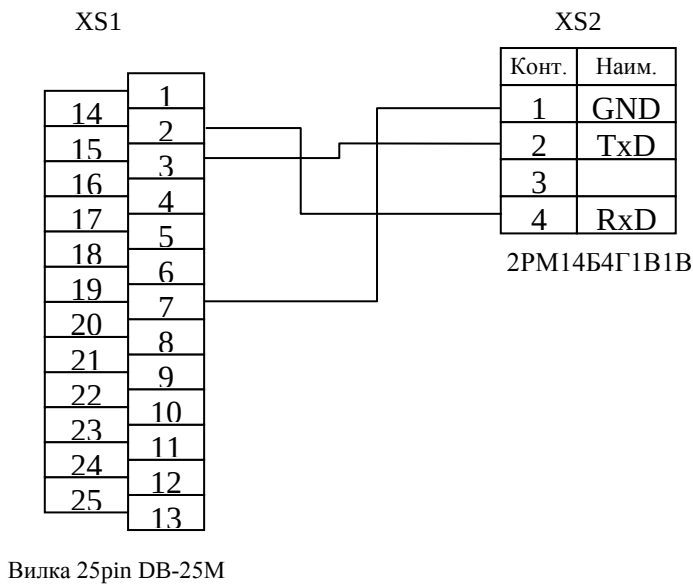
Кабель «БР21-ДН117/ДВ118» (МК101.07.00.0.00-01)
