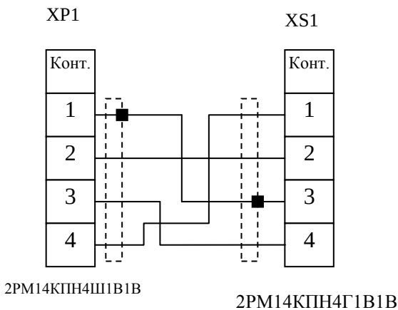
Кабель «БР21-ДН117/ДВ118» (МК101.07.00.0.00-01)
