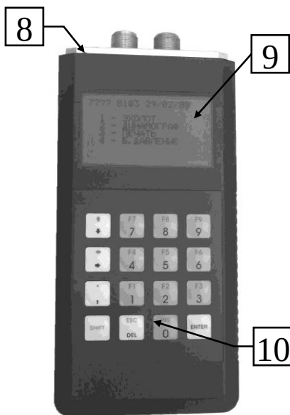
Рис. 3 Верхняя крышка БР
